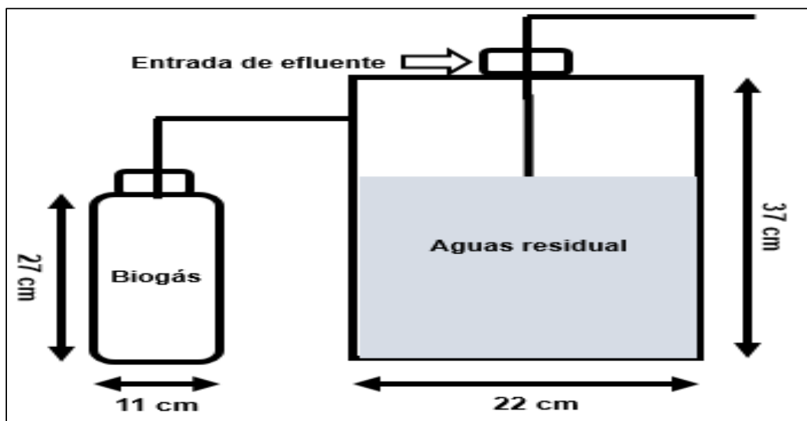
Figura. 5. Biorreactor de capacidad de 10 litros Autor, 2021
