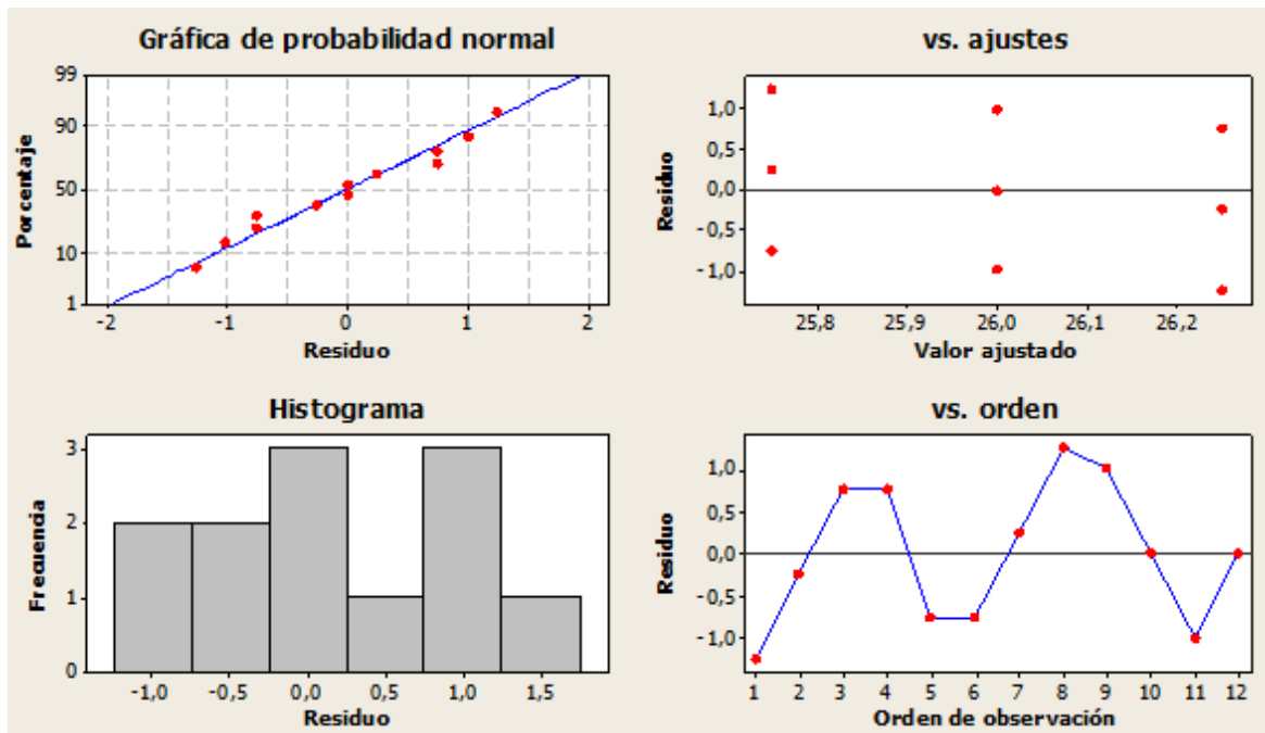
Figura 2. Gráfica de cambio y probabilidad con respecto al parámetro Temperatura. Autor, 2021
