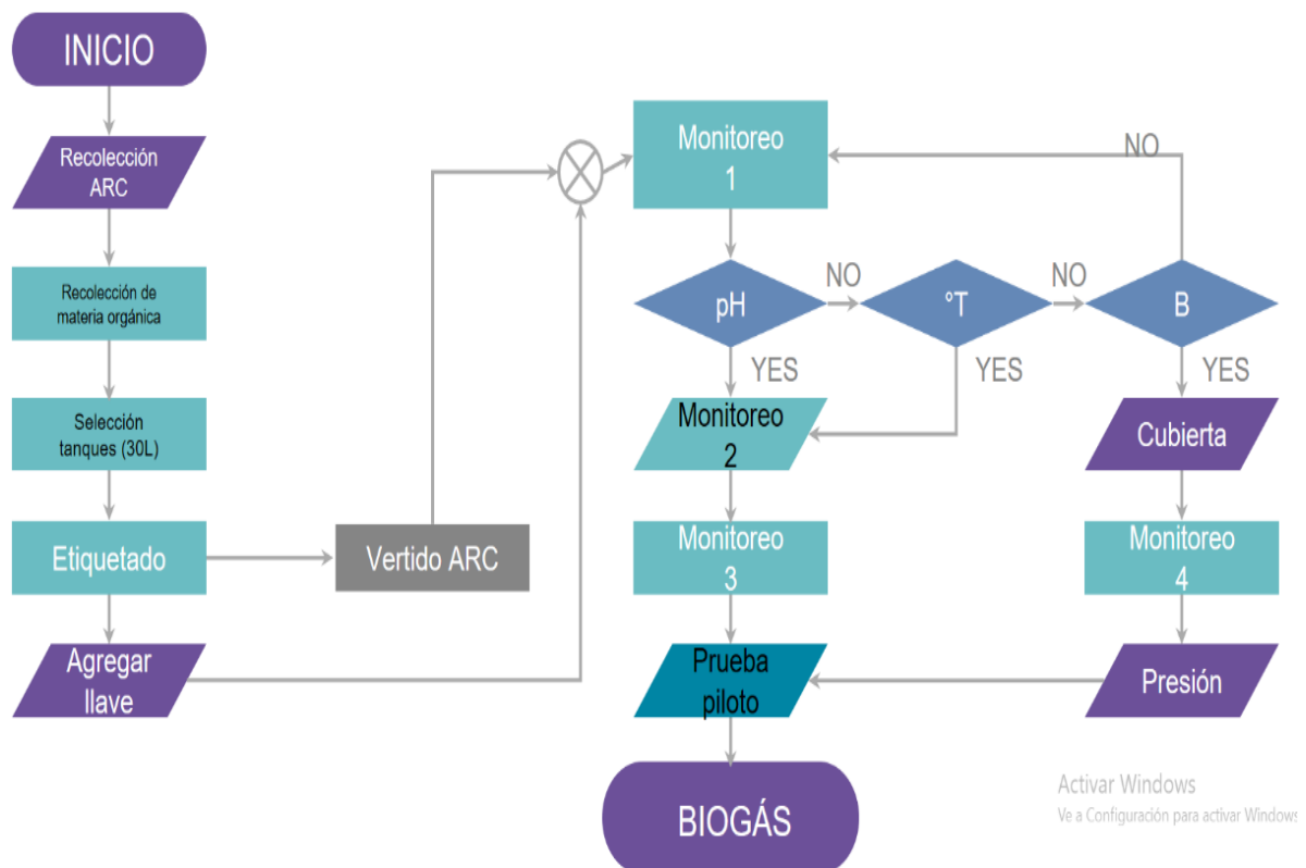
Figura 3. Implementación del biorreactor. Fuente: Autor, 2021
